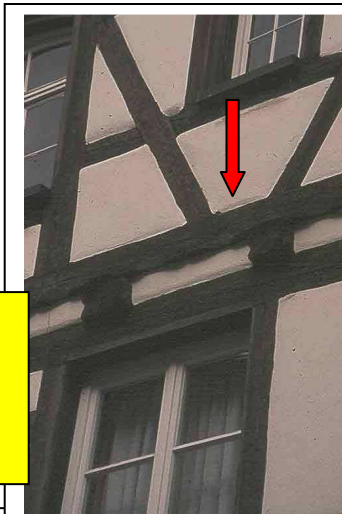
Bild 2: Ein Parallel-Binder, der in einer Fachwerk-Konstruktion die Stockwerksdecke einbindet. Die Deckenbalken werden dabei mit > Schwalbenschwänzen < statisch beweglich gehalten.
