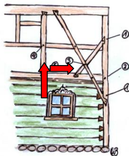
Bild 2: Verwendet werden solche Konstruktionen im Möbelbau, sowie im Holzbau. Rot erkennen wir die Überplattungen im Fachwerkbau.
