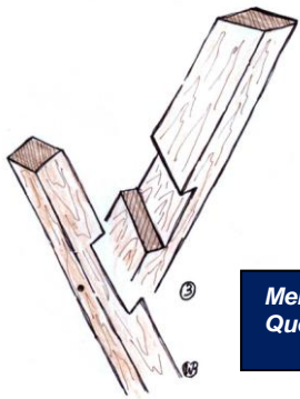
Bild 1: Hier eine Überplattung im Holzbau. Zwei Holzteile werden hälftig eingeschnitten und verbunden.
